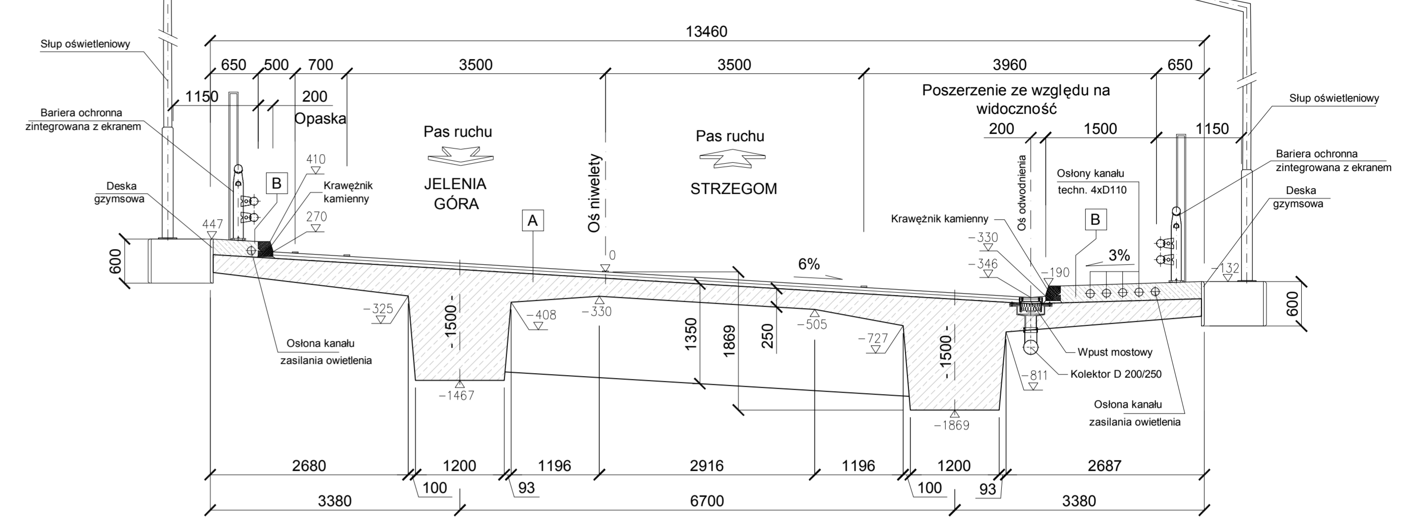
ESTAKADA E1 Przekrój poprzeczny ustroju nośnego Skala 1 : 50
