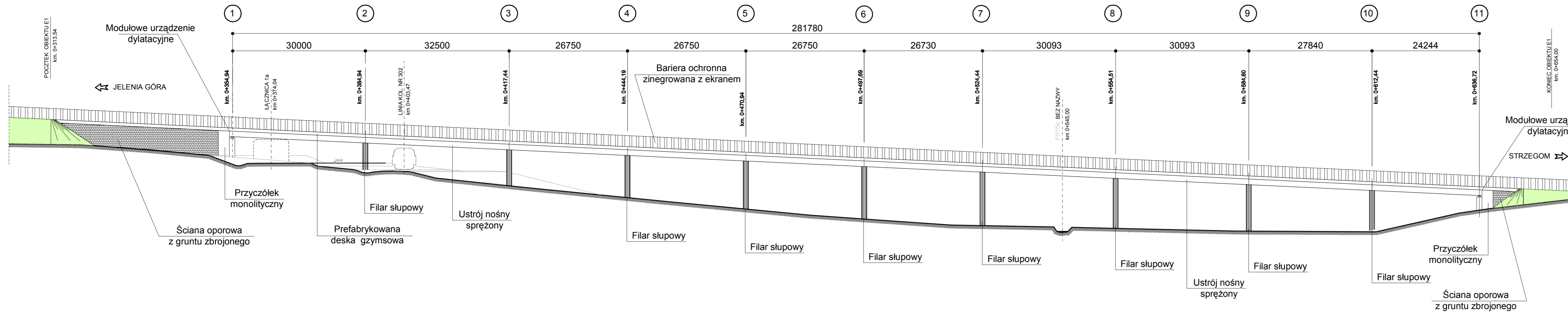
WIDOK Z BOKU - skala 1 : 500
